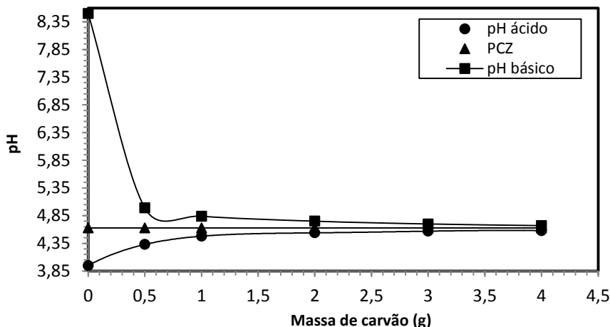
Figura 2. Avaliação do PCZ utilizando-se o método de adição de sólido seco para o carvão sem tratamento partindo-se de 2 pontos, um ácido e outro básico.
