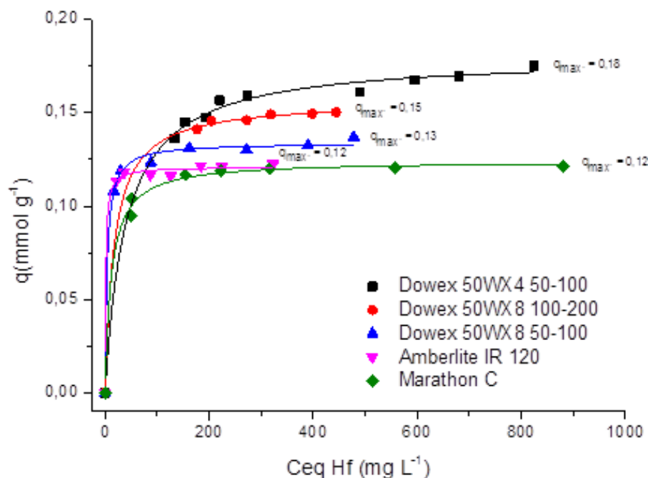
Figura 2. Isoterma de troca iônica para o háfnio. Condições experimentais: T = 28\text{ }^{\circ}\text{C} , agitação = 140\text{ min}^{-1} , [\text{Hf}]_{\text{inicial}} = 5,6 \times 10^{-3}\text{ mol L}^{-1} e [\text{Zr}]_{\text{inicial}} = 7,2 \times 10^{-2}\text{ mol L}^{-1} para a Marathon C; e solução contendo [\text{Hf}]_{\text{inicial}} = 5,5 \times 10^{-3}\text{ mol L}^{-1} e [\text{Zr}]_{\text{inicial}} = 7,4 \times 10^{-2}\text{ mol L}^{-1} para as demais resinas; acidez 1\text{ M HNO}_3 .
