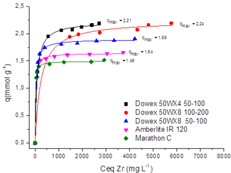
Figura 1. Isoterma de troca iônica para o zircônio. Condições experimentais: T = 28\ ^\circ C , agitação = 140\ min^{-1} , [Zr]_{inicial} = 7,2 \times 10^{-2}\ mol\ L^{-1} e [Hf]_{inicial} = 5,6 \times 10^{-3}\ mol\ L^{-1} para a resina Marathon C e solução contendo [Zr]_{inicial} = 7,4 \times 10^{-2}\ mol\ L^{-1} e [Hf]_{inicial} = 5,5 \times 10^{-3}\ mol\ L^{-1} para as demais resinas, acidez 1\ M\ HNO_3 .
