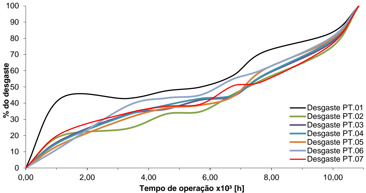
Figura 4. Desgastes pontuais do revestimento na descarga do moinho.
