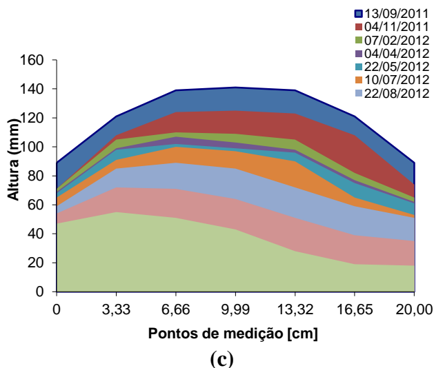
Figura 5. Desgastes do revestimento do moinho: (a) alimentação, (b) centro e (c) descarga do moinho.
