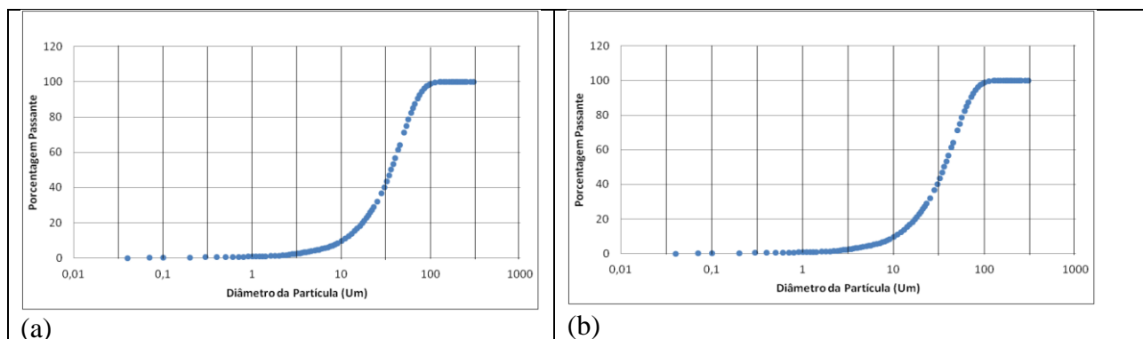
Figura 2. Distribuição granulométrica da amostra de talco lixiviada com ditionito de sódio (a) e ácido clorídrico (b)
